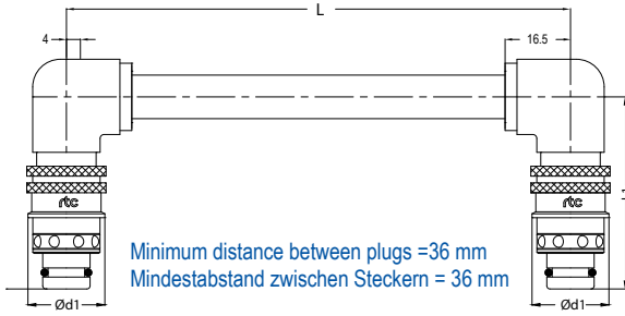
Plug / Stecker
